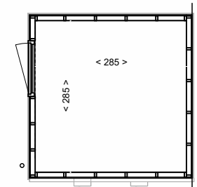
Plattegrond
