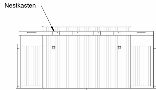
Straatgevel
